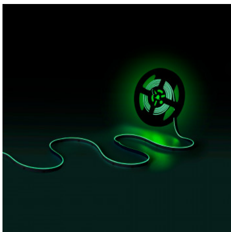
COB RGB LED Strip - 24V DC - Side emission - 12W/m - 10mm - IP20 - 5cm cut - 5 met res roll
